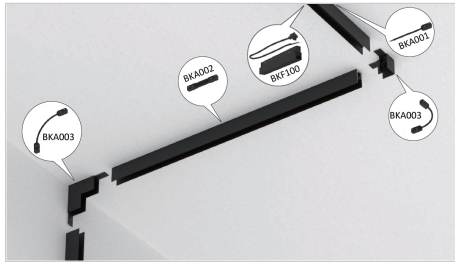
Instalación Conectores
